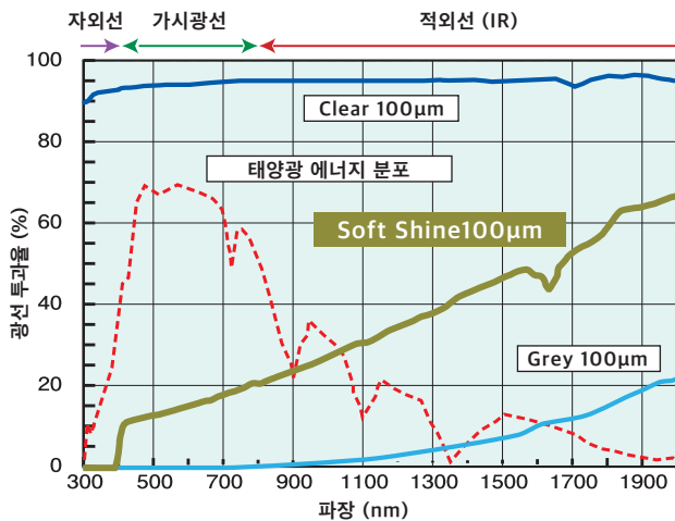
분광 특성(투과율)
