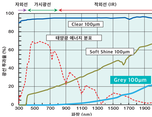
분광 특성(투과율)
