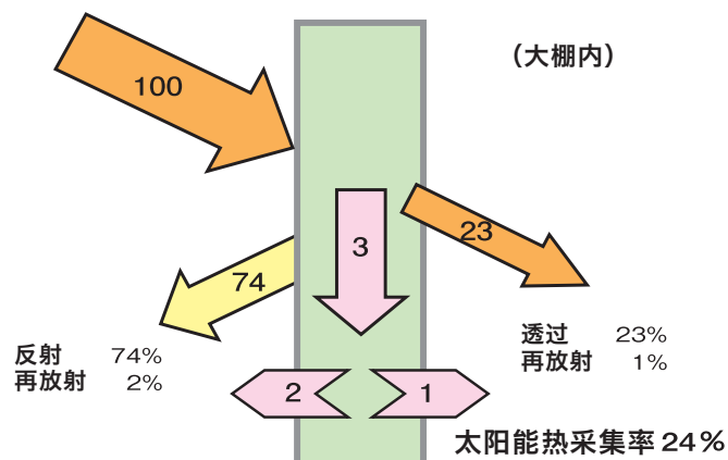
太阳辐射热采集率 (热平衡)
