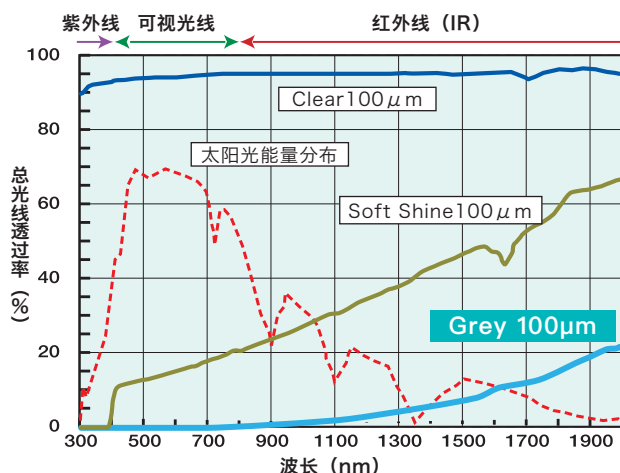
分光特性 (透光率)
