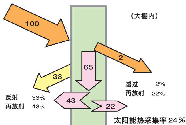
太阳辐射热采集率 (热平衡)
